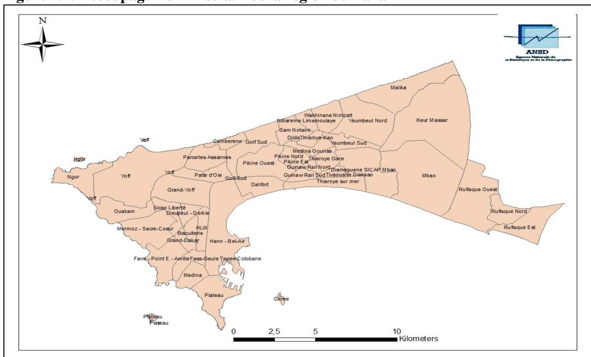
Figure 1.1: Découpage Administratif de la région de Dakar
